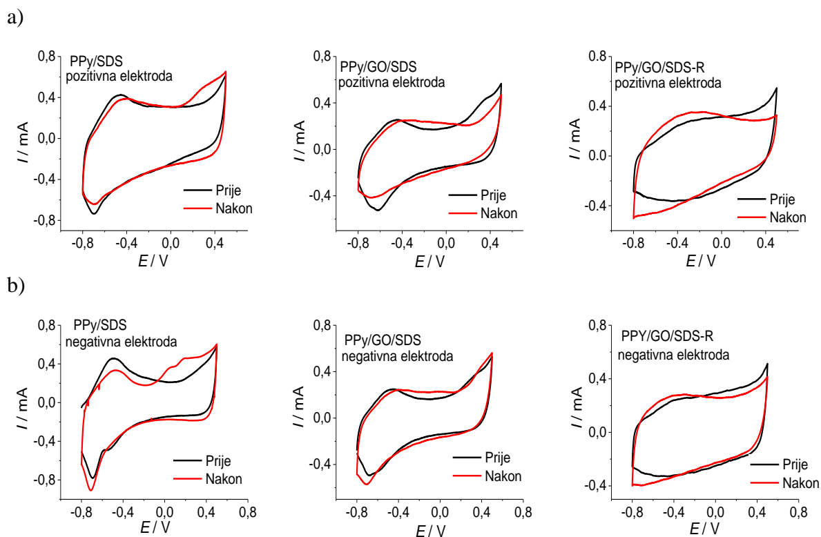
Slika 4.71. Ciklički voltamogrami zabilježeni za slojeve PPy prije i nakon ispitivanja superkondenzatora za a) pozitivnu i b) negativnu elektrodu. Ispitivanja su provedena u 0,5 \text{ mol dm}^{-3} otopini \text{Na}_2\text{SO}_4 , \nu = 50 \text{ mV s}^{-1} .
