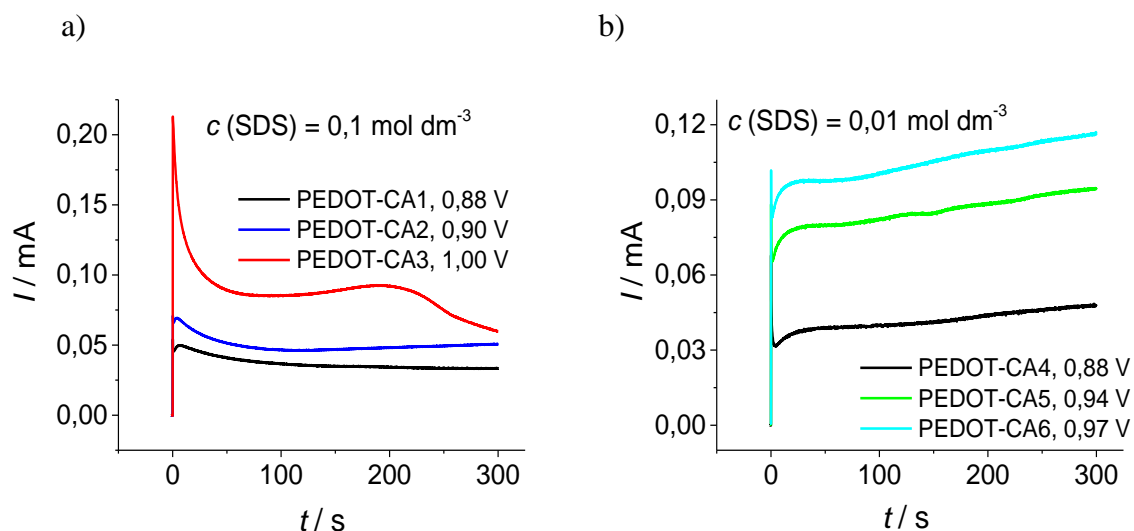
Slika 4.28. Kronoamperometrijski odzivi zabilježeni tijekom sinteze PEDOT slojeva u otopini a) 0,1 mol dm -3 SDS i b) 0,01 mol dm -3 SDS pri različitim vrijednostima potencijala tijekom 300 s, c(\text{EDOT}) = 0,02 \text{ mol dm}^{-3} .
