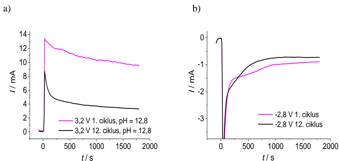
Slika 4.9. Kronoamperometrijski odziv pri a) anodnoj i b) katodnoj polarizaciji pripremljene elektrode u otopini SDS pri pH = 12,8 dobiveni Procedurom 2 .
