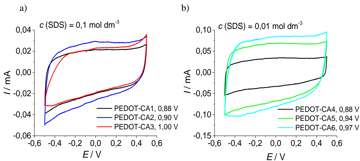
Slika 4.29. Ciklički voltamogrami PEDOT slojeva sintetiziranih u a) 0,1 mol dm -3 i b) 0,01 mol dm -3 otopini SDS, te 0,02 mol dm -3 EDOT pri različitim vrijednostima potencijala u vremenu od 300 s. Ispitivanja su provedena u 0,1 mol dm -3 otopini KCl, \nu = 50 \text{ mV s}^{-1} .
