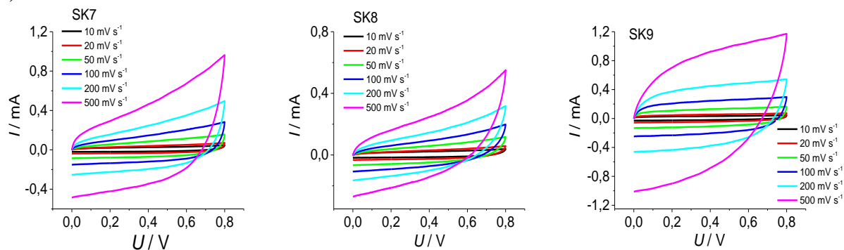
Slika 4.73. Ciklički voltamogrami zabilježeni za SK7, SK8 i SK9 u 0,5 \text{ mol dm}^{-3} otopini \text{Na}_2\text{SO}_4 pri a) v = 50 \text{ mV s}^{-1} prije i nakon punjenja/pražnjenja i b) za različite brzine promjene potencijala.
