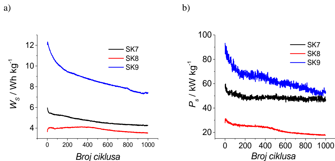
Slika 4.79. Ovisnost a) W_s i b) P_s superkondenzatora o broju ciklusa punjenja/pražnjenja.
