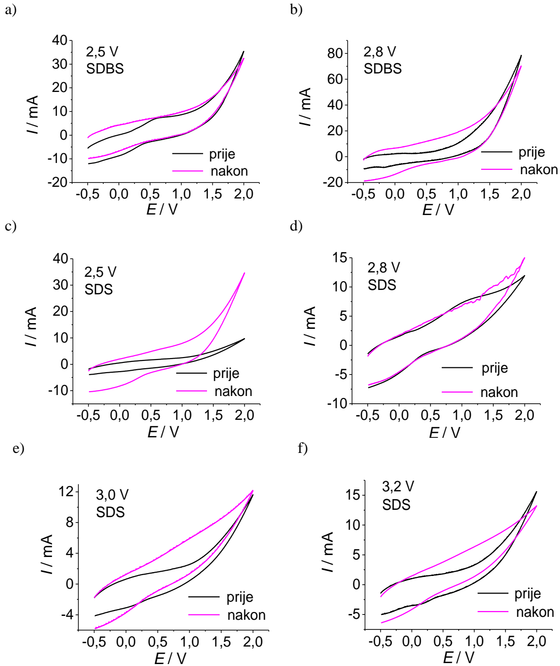
Slika 4.6. Ciklički voltamogrami grafitnog štapića prije i nakon raslojavanja Procedurom 2 pri različitim vrijednostima napona u 0,1 \text{ mol dm}^{-3} otopini a,b) SDBS i c,d,f) SDS.
