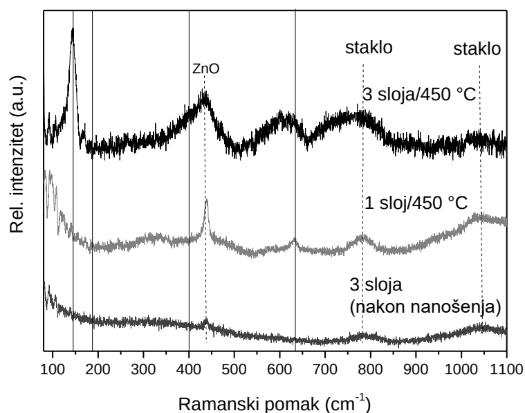
Slika 4.58. Ramanski spektar uzoraka ZnO@TiO 2 dobivenih kemijskom metodom (broj slojeva naglašen na grafu, pune crte označavaju vrpce TiO 2 anatas).
