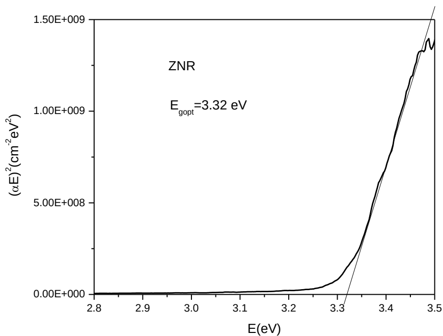
Slika 4.62. Određeni energijski procijep ZNR iz grafičkog prikaza (\alpha E)^2 nasuprot energiji fotona E ; linija predstavlja fit za vrijednost n = \frac{1}{2} [133].
