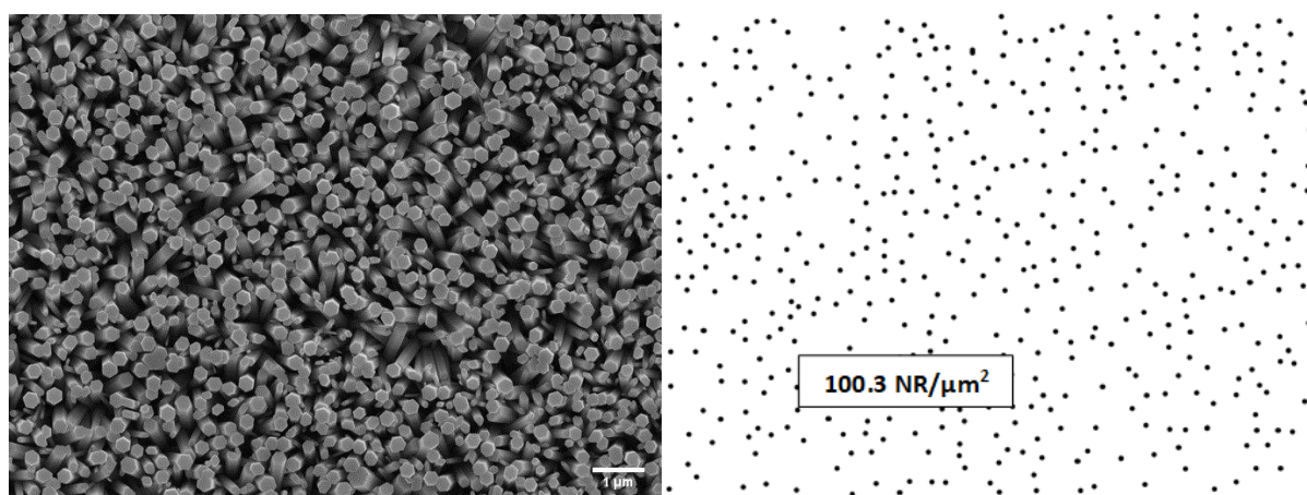
Slika 4.11. SEM mikrografija ZnO nanoštapića s prikazom tipične površinske po kvadratnom mikrometru (uvjeti reakcije 0,125 M; 90 °C, 60 min).
