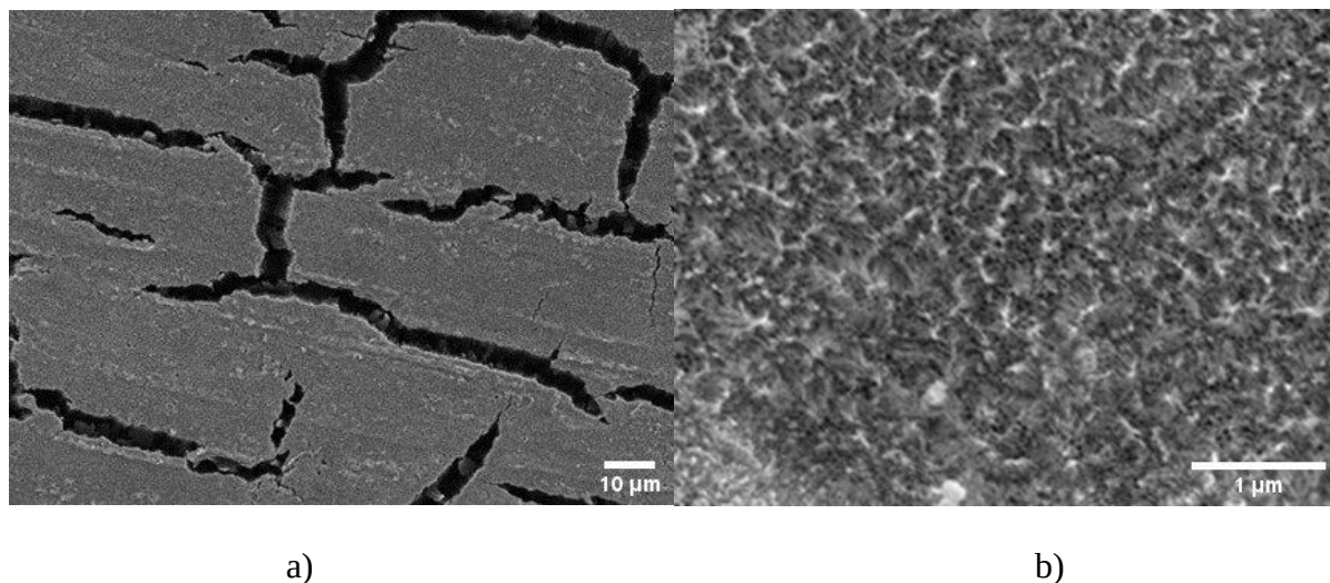
Slika 4.27. SEM mikrografije \text{TiO}_2 NT s različitim udjelima vode u elektrolitu: a) i b) 2 %, c) i d) 6 %, e) i f) 12 %, g) i h) 18 % te i) i j) 24 %.
