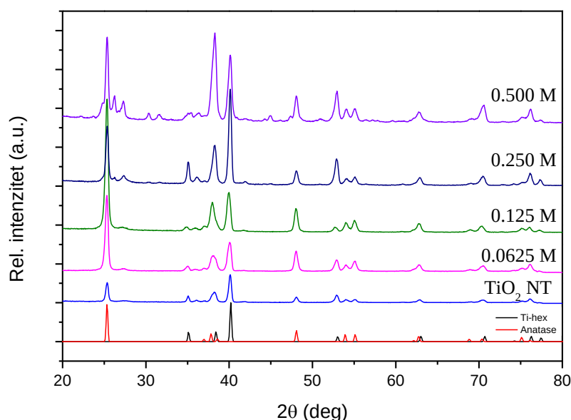
Slika 4.37. GIXRD difraktogrami za uzorke nemodificiranog TiO 2 NP i Cu modificirane TiO 2 NP.
