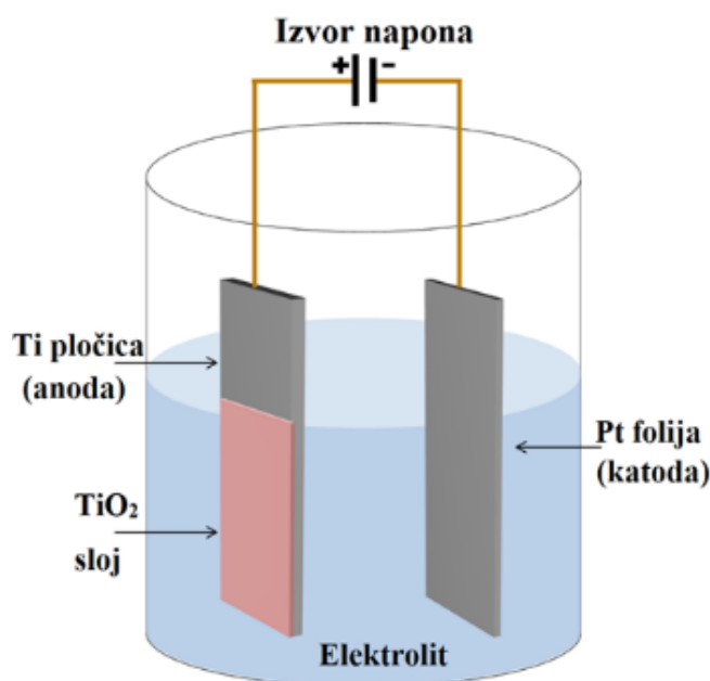
Slika 2.12. Shematski prikaz elektrokemijske ćelije za sintezu \text{TiO}_2 NT anodizacijom Ti [75].
