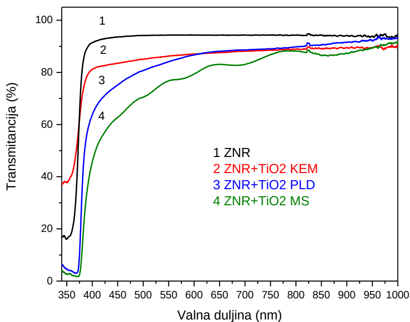
Slika 4.61. Transmitancija ZnO@TiO 2 kompozita, za uzorke dobivene: 1 sloj kemijskim nanošenjem ; 7500 pulseva u vakuumu; magnetronsko rasprašenje 30 min [133].
