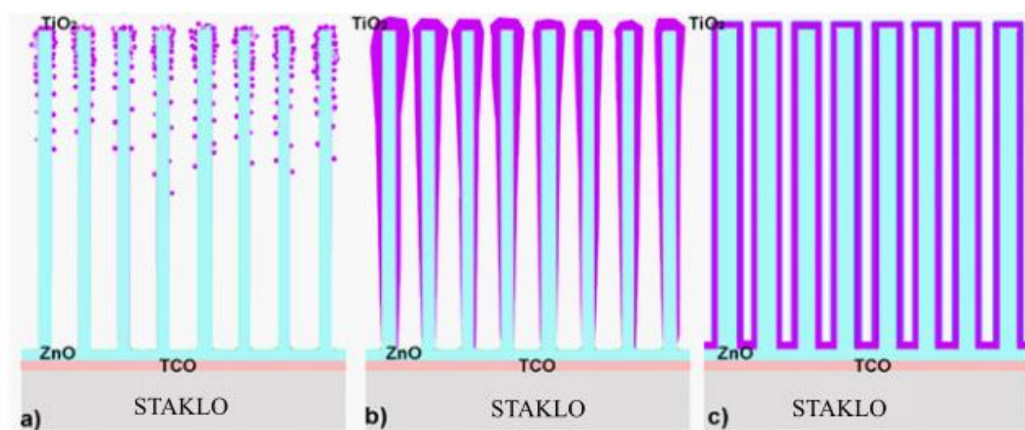
Slika 4.41. Shematski prikaz TiO 2 slojeva s različitim morfologijama: a) TiO 2 sloj u obliku nanočestica raznih veličina; b) sloj TiO 2 sa zadebljanim vrhovima nanoštapića; c) glatki, homogeni sloj TiO 2 [133].
