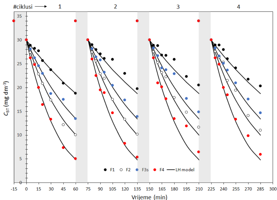
Slika 4.40. Kinetika razgradnje BT na uzorcima iz serije modificirane SC tehnikom [132].
