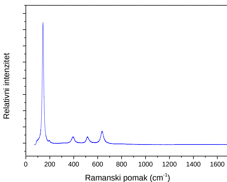
Slika 4.29. Ramanski spektar \text{TiO}_2 NT pripremljenih s udjelom vode 12 % nakon grijanja na 450^\circ\text{C} .
