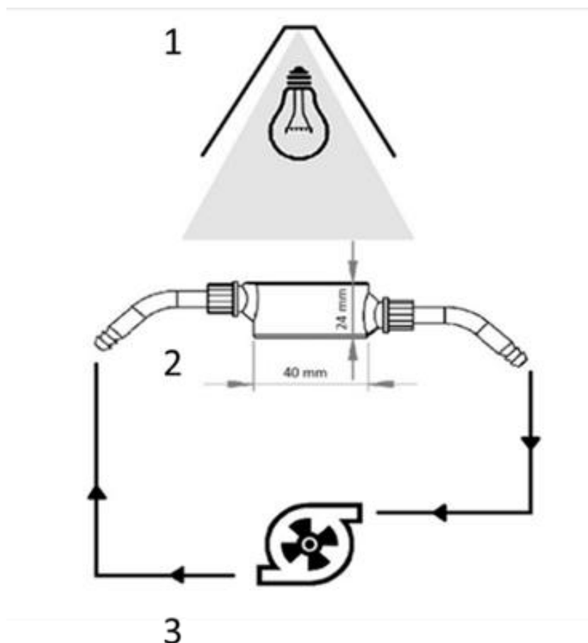
Slika 3.4. Shematski prikaz reaktora: 1 izvor zračenja, 2 protočna ćelija ( V = 30 ml), 3 peristaltička pumpa.
