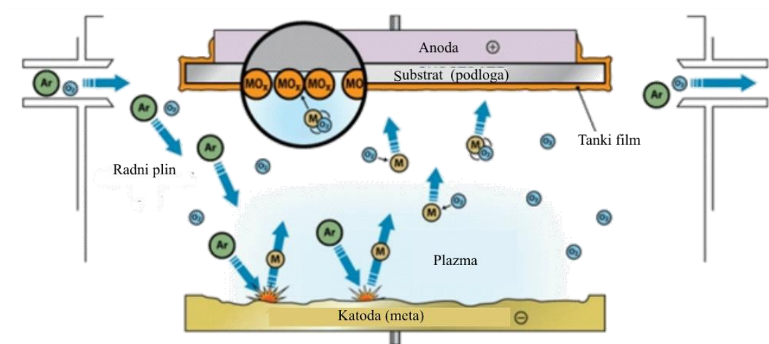
Slika 2.14. Shematski prikaz magnetronskog rasprašenja [89].
