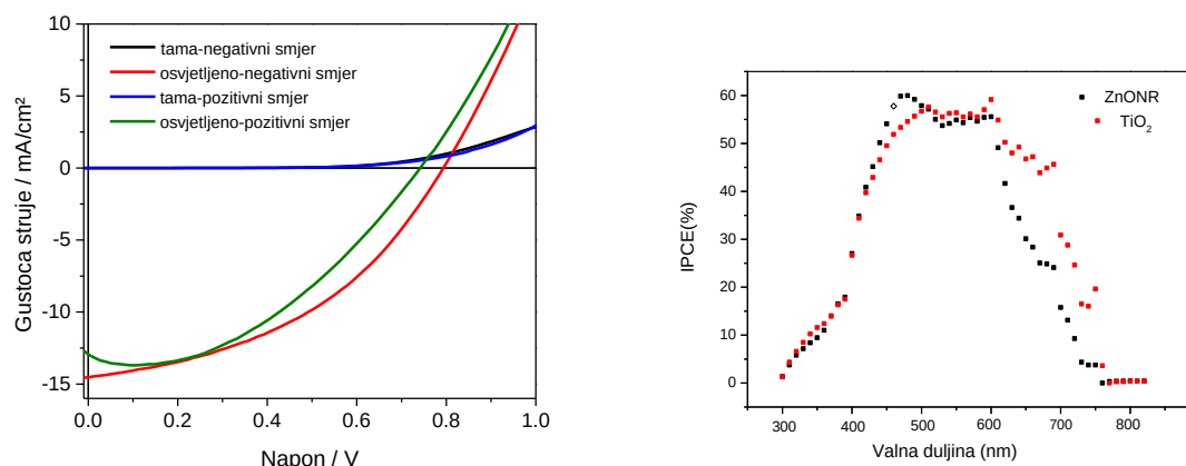
Slika 4.24. J-V karakteristika PSC s ZNR ETL slojem, b)EQE spektar PSC s \text{TiO}_2 i ZNR ETL slojem.
