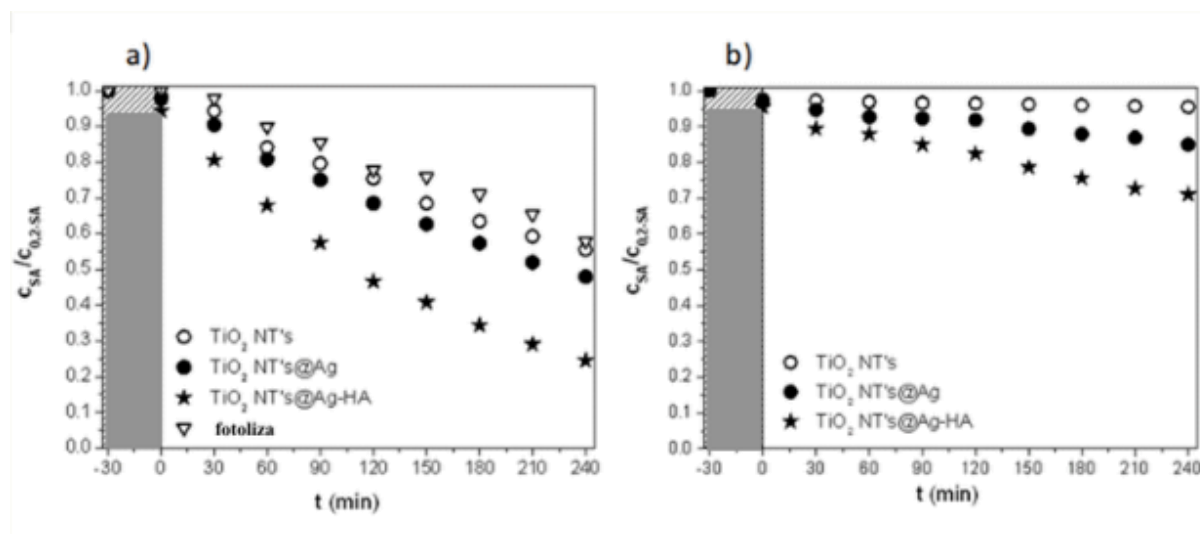
Slika 4.32. Kinetika fotolize i fotokatalitičke razgradnje SA: a) pod osvjetljenjem punog spektra b) pod osvjetljenjem vidljivog dijela spektra; C_{0,SA} = 0,2 \text{ mmol dm}^{-3} , pH 4. Sivi dio označava adsorpciju u mraku potrebnu za postizanje ravnoteže [131].
