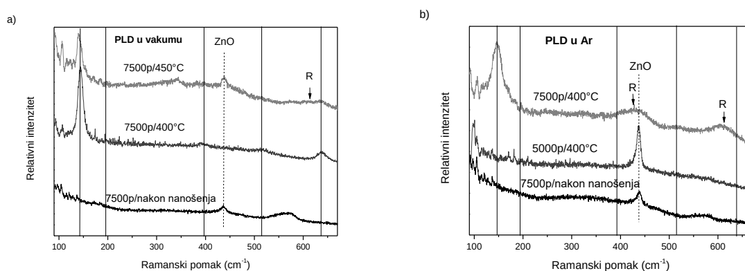
Slika 4.45. Ramanski spektar \text{TiO}_2 nanesenog PLD om: a) u vakuumu, b) u argonu. Puncne crte označavaju vrpce anatas \text{TiO}_2 , dok R označava rutilne vrpce.
