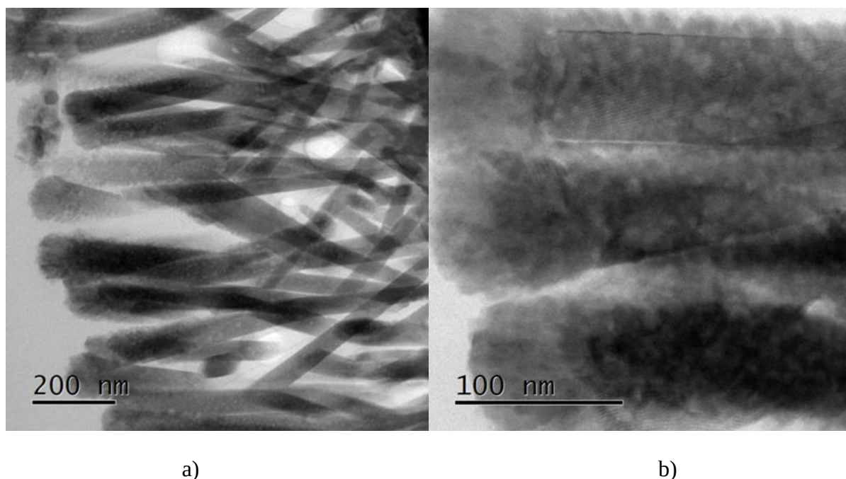
Slika 4.50. TEM mikrografija ZnO@TiO 2 uzoraka dobivenih MS u trajanju od 60 min.
