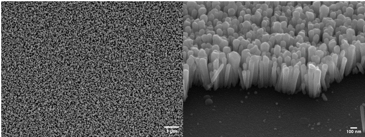
Slika 4.42. SEM mikrografija uzorka ZnO@TiO 2 dobivenog korištenjem 5000 pulseva u 30 Pa Ar.
