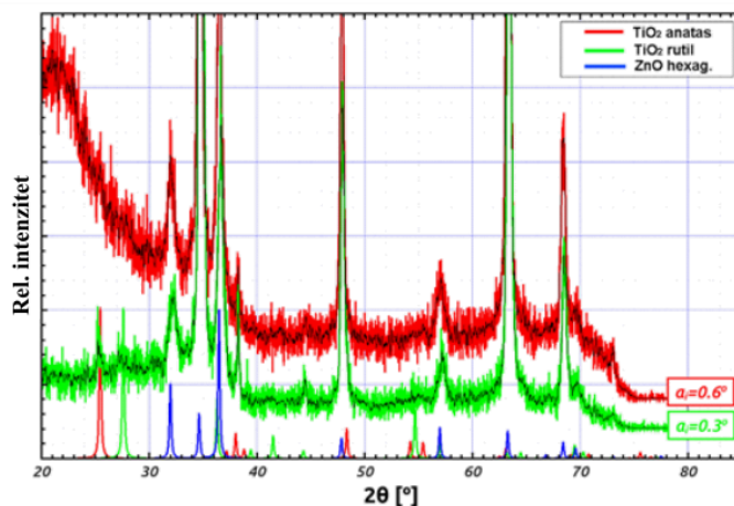
Slika 4.46. GIXRD difraktogrami \text{ZnO@TiO}_2 PLD uzoraka [133].
