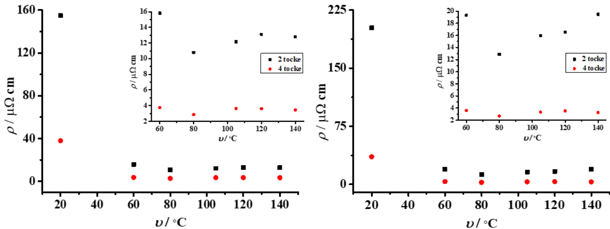
Slika 75. Grafički prikaz otpornosti nanosrebrnih elektroda širina 1 mm ( lijevo ) te 2 mm ( desno ) o temperaturi sinteriranja u trajanju od 20 min, prema podacima iz tablice 9 . Umetak: uvećani dio početnog dijela grafičkog prikaza.
