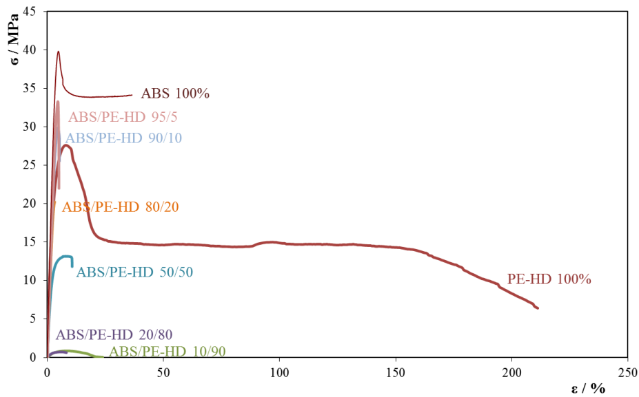
Slika 34. Grafički prikazi ovisnosti naprežanja o istezanju za ABS i polimerne mješavine s PE-HD-om pripravljene u ekstruderu
