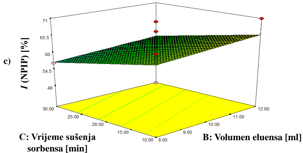
Slika P5. Trodimenzionalni prikazi odzivnih površina za NPIP
