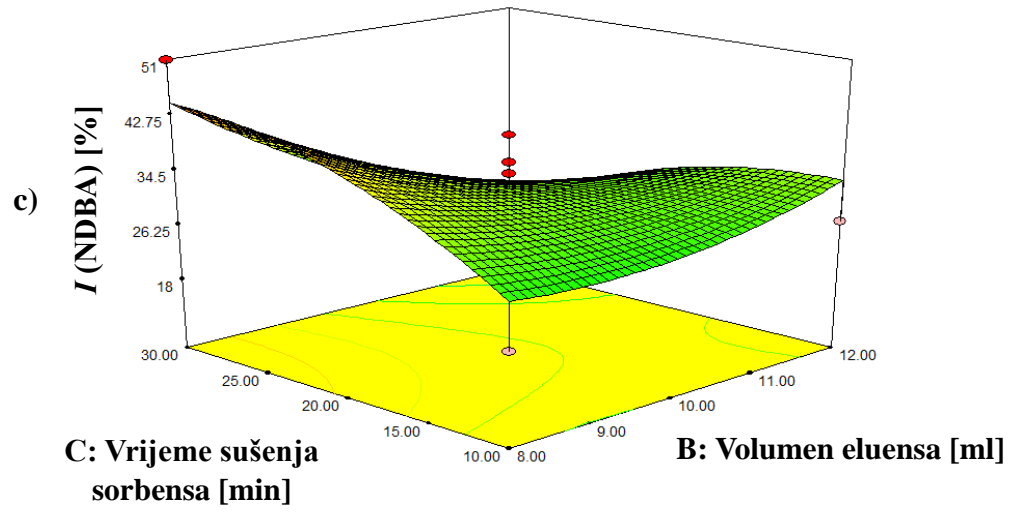
Slika P7. Trodimenzionalni prikazi odzivnih površina za NDBA
