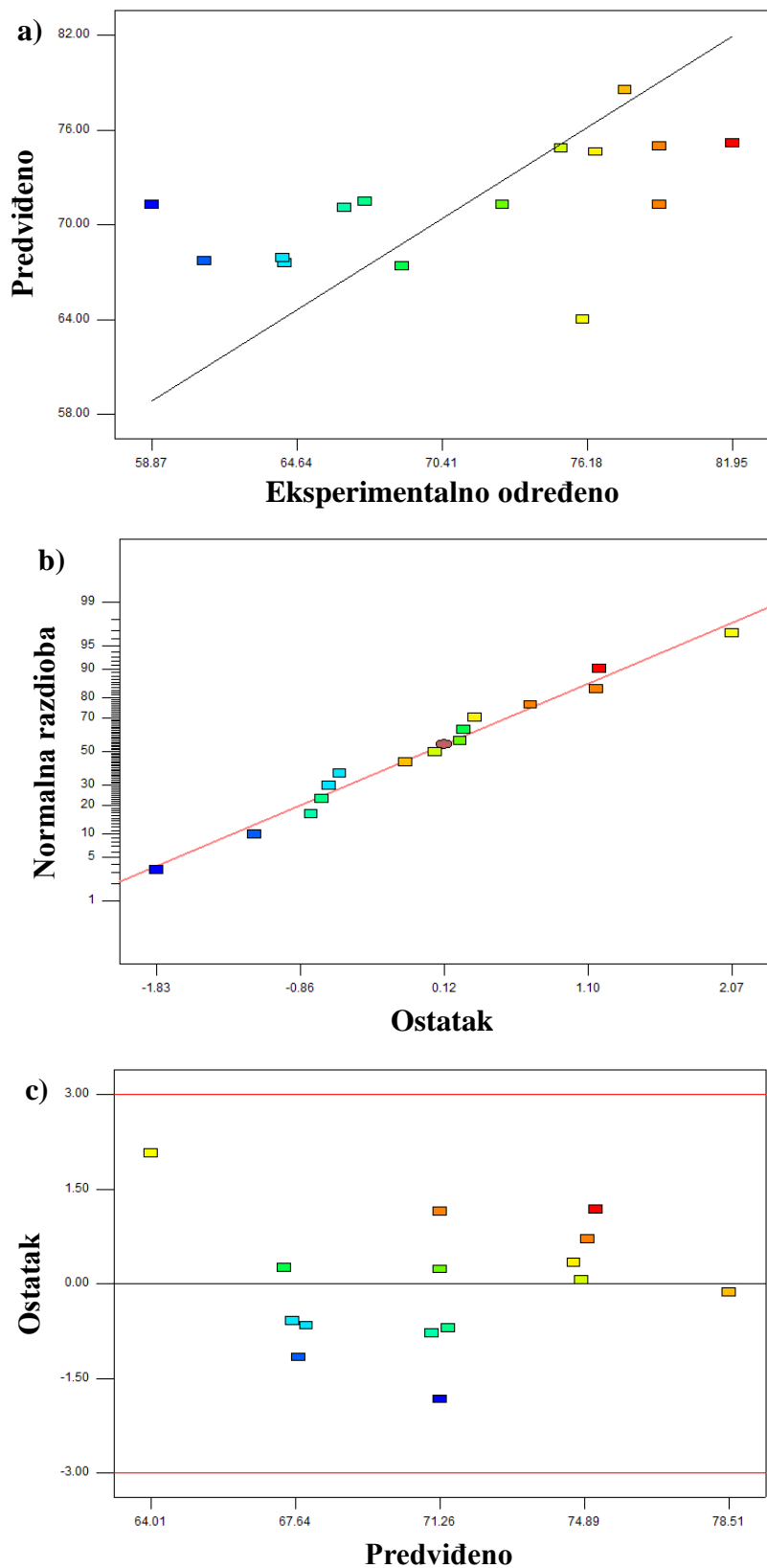
Slika 28. Grafička procjena valjanosti modela, dijagnostička analiza ostatka za NPYR
