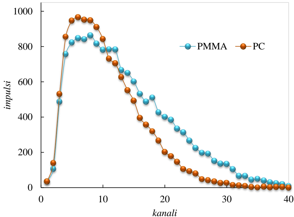
Slika 55. Spektar ^{90}\text{Y} dobiven Čerenkovljevim zračenjem ( A \sim 15 Bq) otopine izotopa u kolonama izrađenima od pleksiglasi (PMMA) i polikarbonatnog (PC) materijala.
