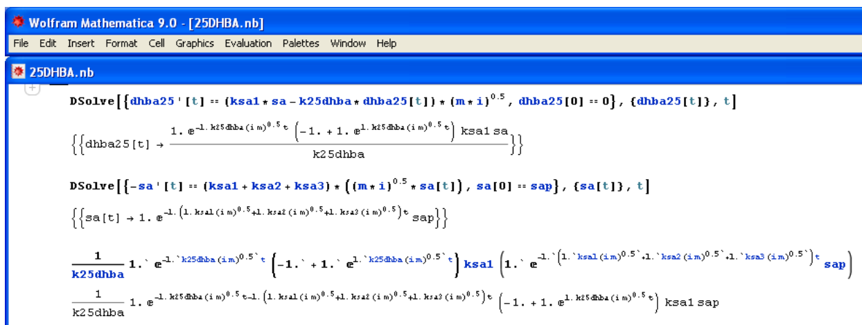
Slika P.3. Prikazuje rješenje matematičkog modela koji opisuje razgradnju 2,5-DHBA u fotoreaktoru R1 s imobiliziranim TiO 2 uz UV-A zračenje. Koncentracija 2,5-dhba u vremenu t (dhba25[t]), konstanta brzine razgradnje SA u 2,5-DHBA (ksa1), konstanta brzine razgradnje SA u 2,3-DHBA (ksa2), konstanta brzine razgradnje SA u ostale nusprodukte (ksa3), koncentracija SA u vremenu t (sa), početna koncentracija SA (sap), konstanta razgradnje 2,5-DHBA na ostale nusprodukte (k25dhba), apsorpcijski koeficijent (m), fluks upadnog zračenja (i)
