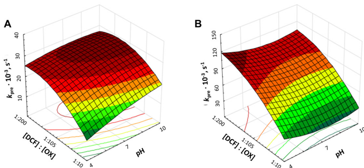
Slika 11. Prikaz utjecaja procesnih parametara na kinetiku razgradnje DCF UV-C/H 2 O 2 (A) i UV-C/S 2 O 8 2- (B) procesima.
