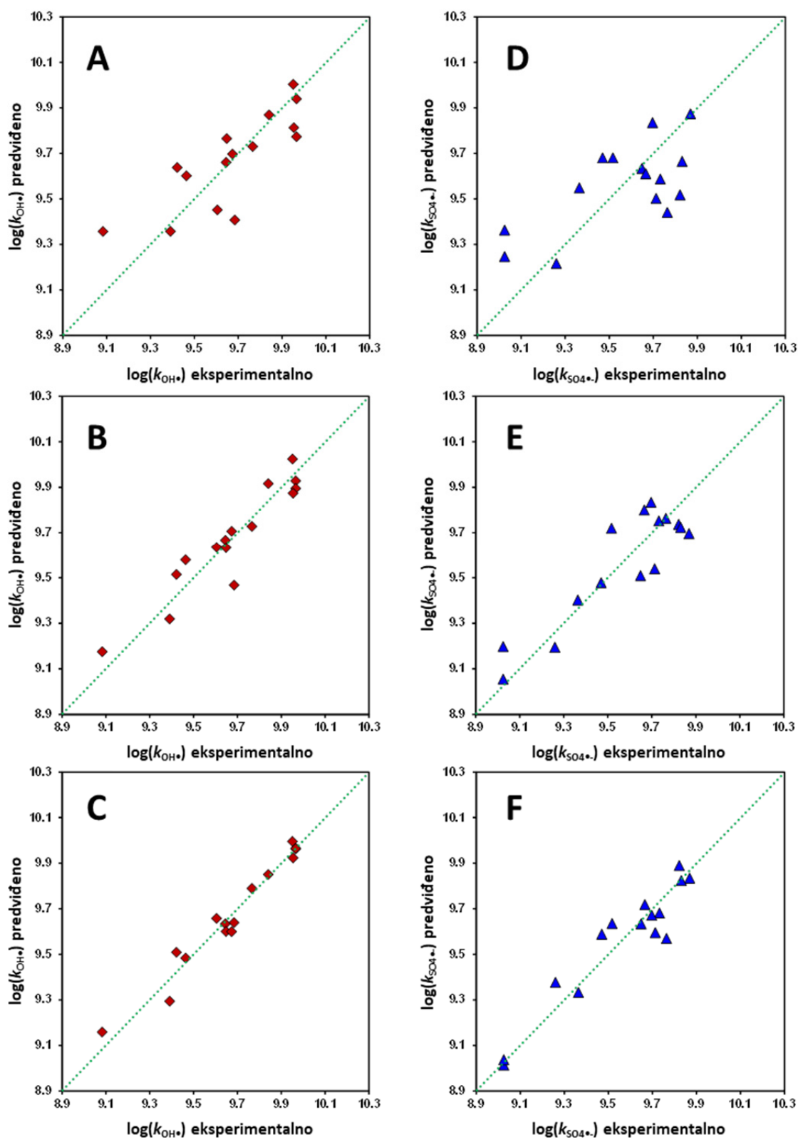
Slika 37. Točnost razvijenih 1- (A i D), 2- (B i E) i 3-parametarskih (C i F) QSAR modela kinetike razgradnje UV-C/H 2 O 2 (crveno) i UV-C/S 2 O 8 2- (plavo) procesa oksidacije.
