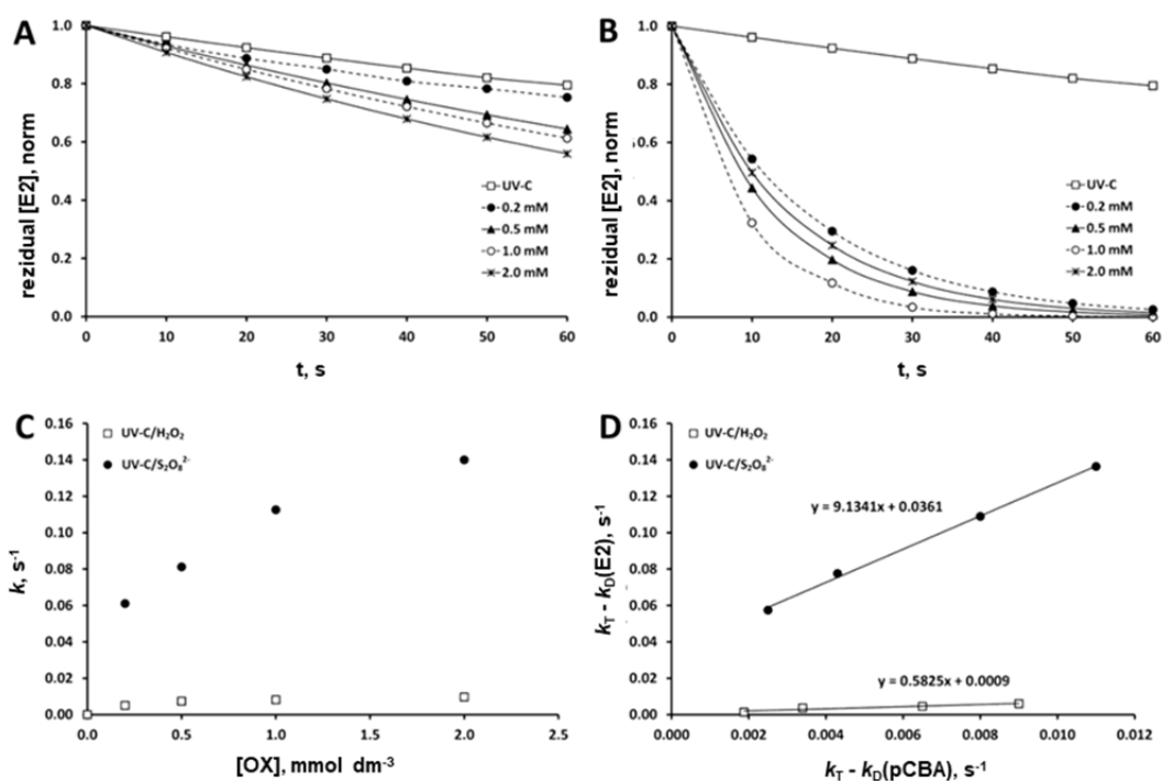
Slika 31. Određivanje kinetike drugog reda E2: A) razgradnja UV-C/ \text{H}_2\text{O}_2 procesom, B) razgradnja UV-C/ \text{S}_2\text{O}_8^{2-} procesom, C) kinetika pseudo prvog reda za oba procesa, D) određivanje kinetike drugog reda.
