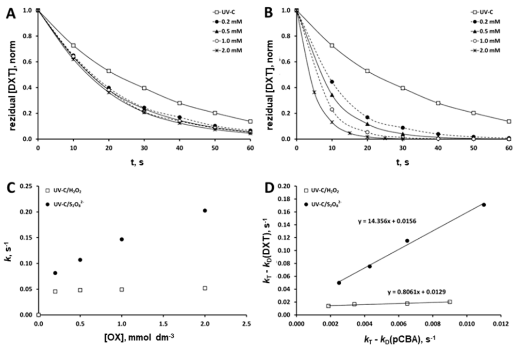
Slika 30. Određivanje kinetike drugog reda DXT: A) razgradnja UV-C/ \text{H}_2\text{O}_2 procesom, B) razgradnja UV-C/ \text{S}_2\text{O}_8^{2-} procesom, C) kinetika pseudo prvog reda za oba procesa, D) određivanje kinetike drugog reda.
