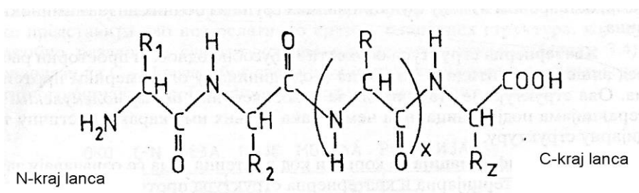
Slika 2. Peptidni lanac [13]
