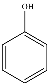
Slika 3.1. Kemijska struktura fenola
