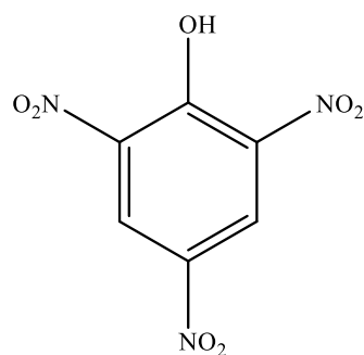
Slika 3.2. Kemijska struktura pikrinske kiseline ili 2,4,6-trinitrofenola
