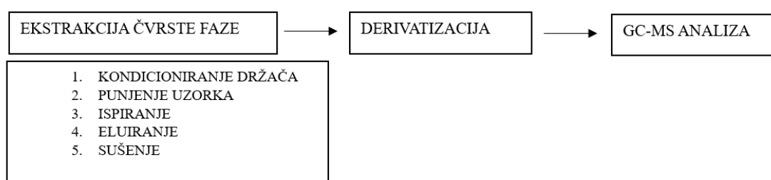
Slika 3.18. Analitički postupak analize fenola i klorfenola
