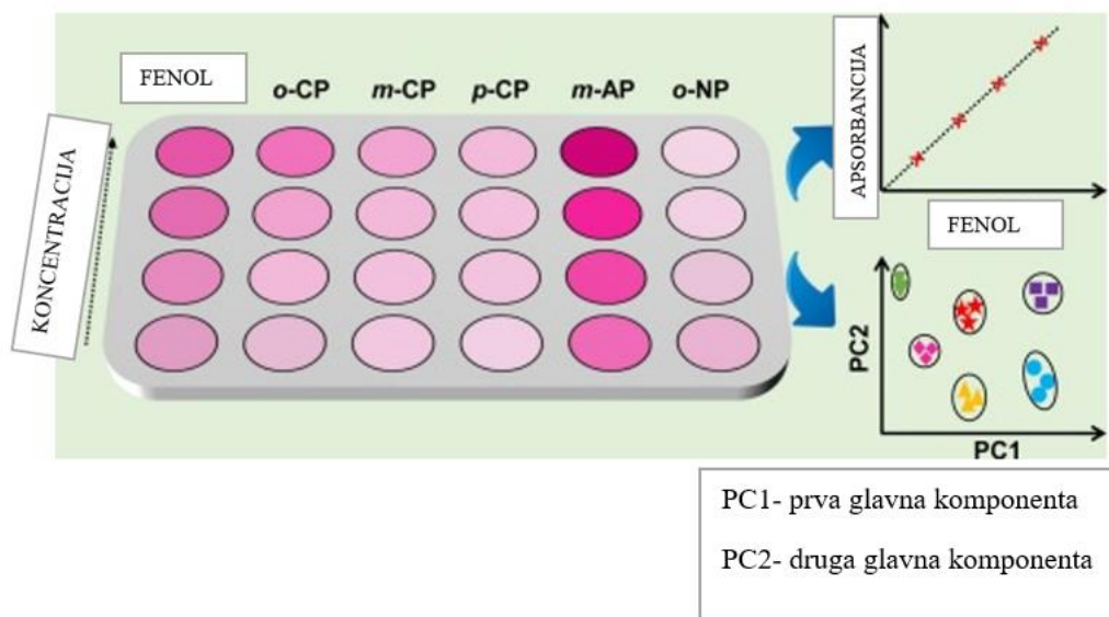
Slika 3.14. Kolorimetrijska kvantifikacija fenolnih onečišćivala
