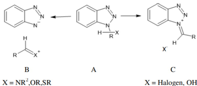
Slika 2. Shematski prikaz ionizacije spojeva s R i heteroatomom 25 .
