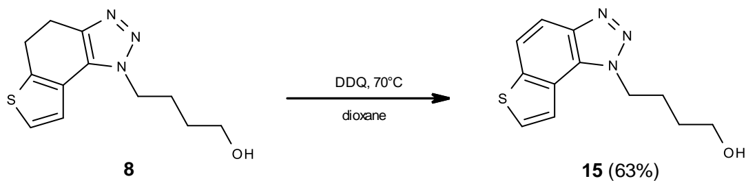
Shema 19. Sintaza 4-(1H-tieno[3',2':3,4]benzo[1,2-d][1,2,3]triazol-1-il)butan-1-ola ( 15 ).
