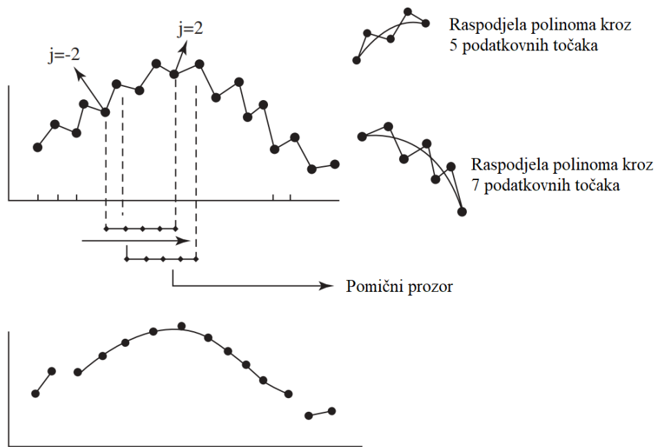
Slika 15. Savitsky-Golay filter s veličinom prozora od 2M + 1 = 5 točaka ( M=2 ). Umjesto prosjeka podatkovnih točki u pokretnom prozoru, koristi se tehnika prilagođavanja polinoma. Gornja slika prikazuje izvorni signal, a donja izgladjeni, tj. obrađeni signal. [13]
