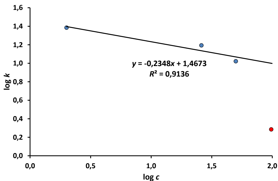
Slika 38. Model pravca kod sukroze dobiven na temelju log k vrijednosti predviđenih QSRR modelom, s izuzetom vrijednosti pri 98 mM KOH (crvena točka).
