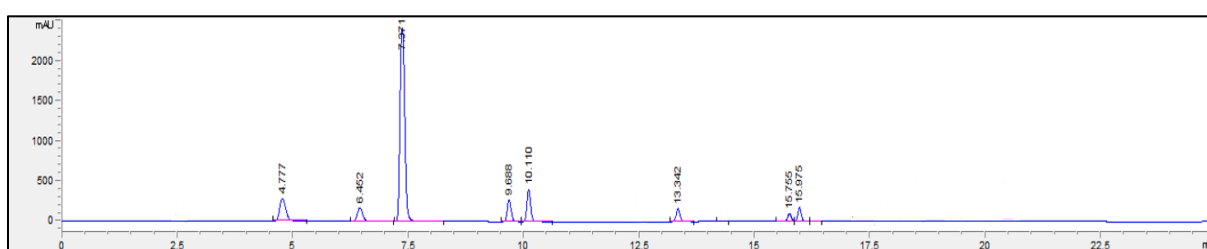
Slika 44. Kromatogram dobiven za četvrti gradijent
