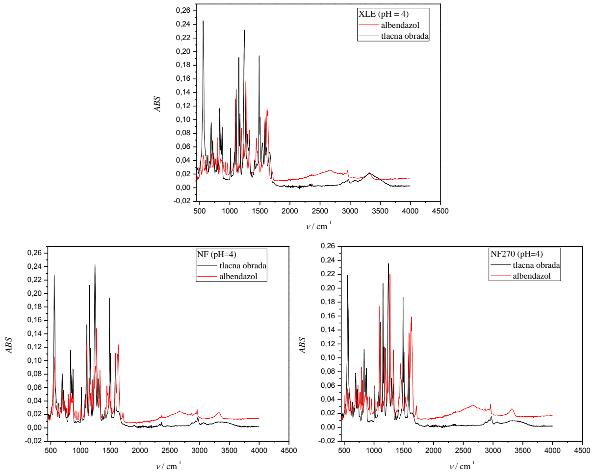
Slika 4.10. FTIR spektar za XLE, NF, i NF270 membrane nakon tlačne obrade i tretmana otopinom albendazola.
