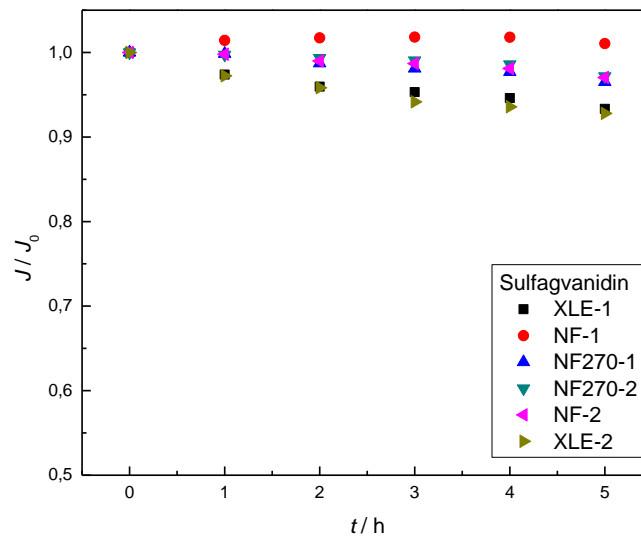
Slika 4.1. Ovisnost normaliziranog fluksa permeata o vremenu.
