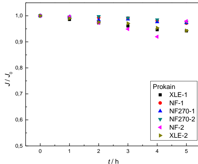
Slika 4.7. Ovisnost normaliziranog fluksa permeata o vremenu.
