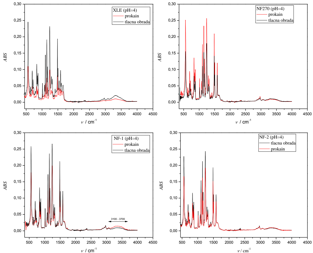
Slika 4.3. FTIR spektrar za XLE, NF-1, NF-2 i NF270 membranu nakon tlačne obrade i tretmana otopinom prokain·HCl.
