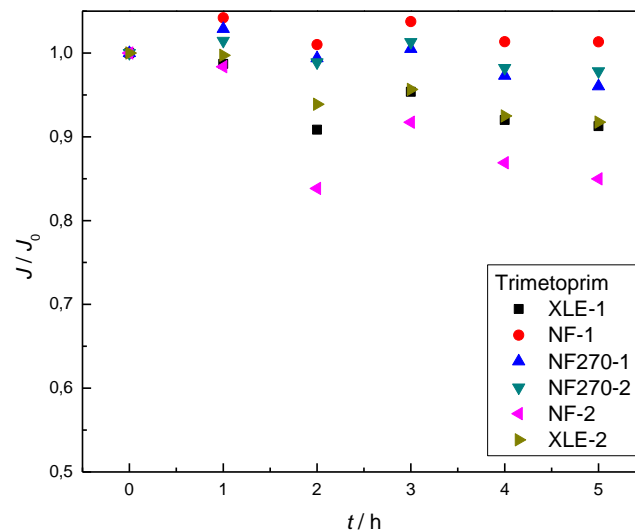
Slika 4.3. Ovisnost normaliziranog fluksa permeata o vremenu.
