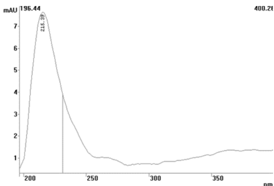
Slika 110. Apсорpcijski spektar razgradnog produkta ( t_R=21,227 min) acetamiprida koji je nastao tijekom fotolize otopine acetamiprida uz prisutnost natrijevog hipoklorita
