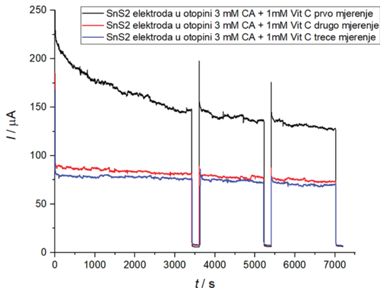
Slika 4.16. Rezultati dobiveni fotoelektrokemijskim procesom za SnS 2 elektrodu u otopini 3 mM kofeinske kiseline i 1 mM vitamina C u 0.1 M NaCl prilikom tri mjerenja
