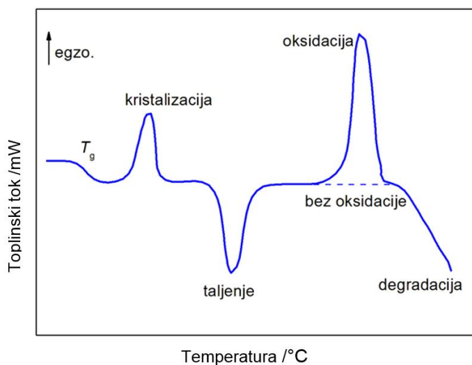
Slika 12. DSC krivulja polimera s mogućim faznim prijelazima [31]
