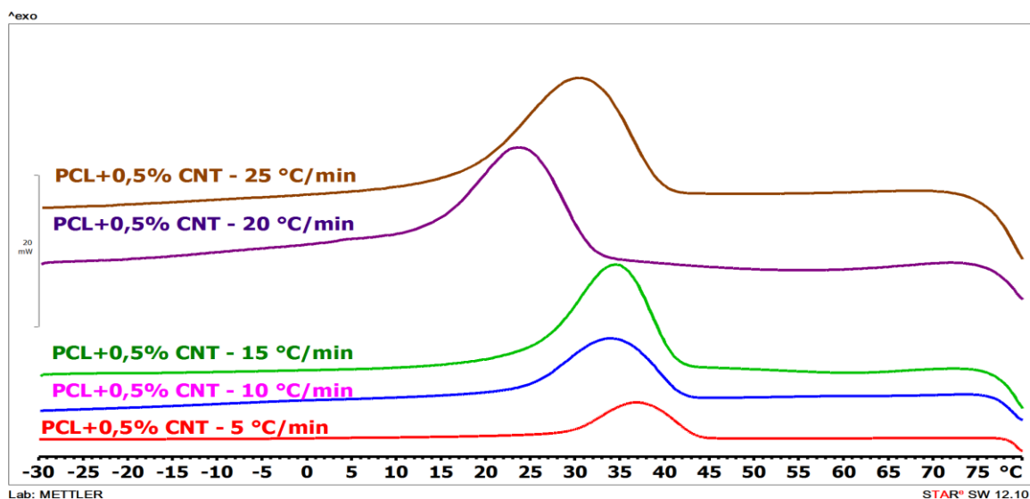
Slika 14. DSC krivulje nakon 2.ciklusa hlađenja za PCL i PCL/CNT nanokompozite s udjelom 0,2 i 0,5 mas.% CNT pri različitim brzinama zagrijavanja.
