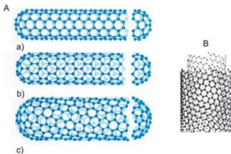
Slika 3. A - Shematski prikaz zamotavanja heksagonskih grafenskih listova u nanocjevčice različitih morfologija: a) fotelja, b) cik-cak, c) kiralna; B - shematski prikaz višestijene nanocjevčice (MWCNT). [1]
