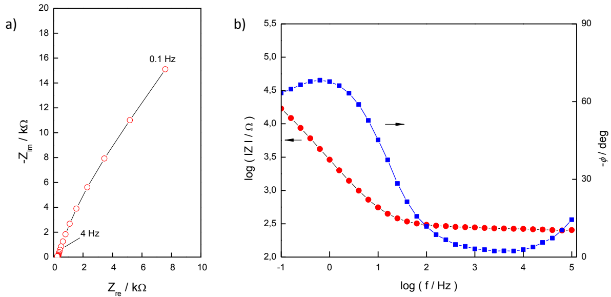
Slika 4.2.3.4. Prikaz EIS rezultata dobivenih za Pt elektrodu na koju je nanesen rGO(OMW, pH=10) pri potencijalu -200 mV a) Nyquistov dijagram, b) Bodeov dijagram
