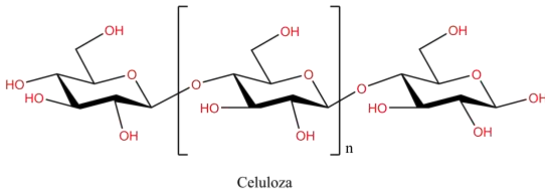
Slika 2.28. Struktura celuloze [282]
