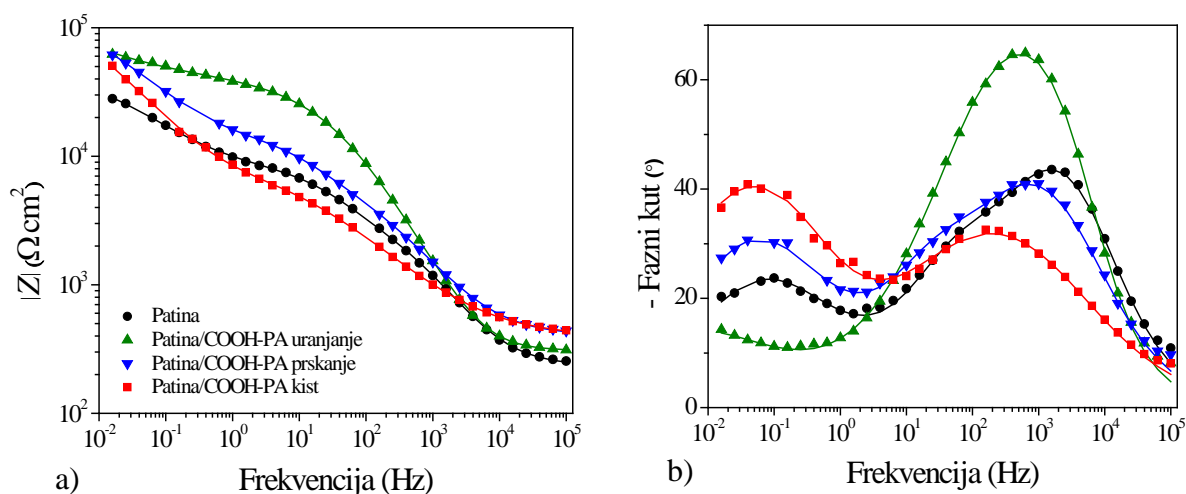
Slika 4.53. EIS – Bodeov prikaz za nezaštićeni uzorak i uzorke zaštićene filmom COOH-PA nakon dva tjedna uranjanja u kiselu kišu: a) modul impedancije i b) fazni kut (simboli – eksperimentalni podaci, linije – rezultati dobiveni korištenjem modela prikazanog na slici 4.54.). 82
