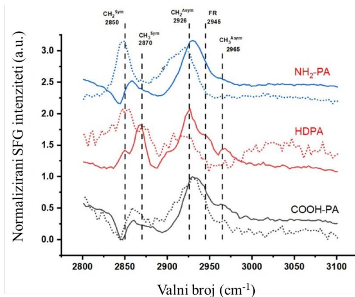
Slika 4.15. SFG spektralizirani intenziteti (a.u.) u funkciji valnog broja (cm -1 ) za 0,1 mM (isprekidana linija) i 1 mM (puna linija) NH 2 -PA, HDPA i COOH-PA na bronci. Vertikalne linije predstavljaju odgovarajuće vrhove. 81
