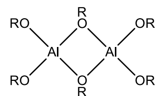
Slika 18. Struktura dimernog aluminijeva alkoksida
