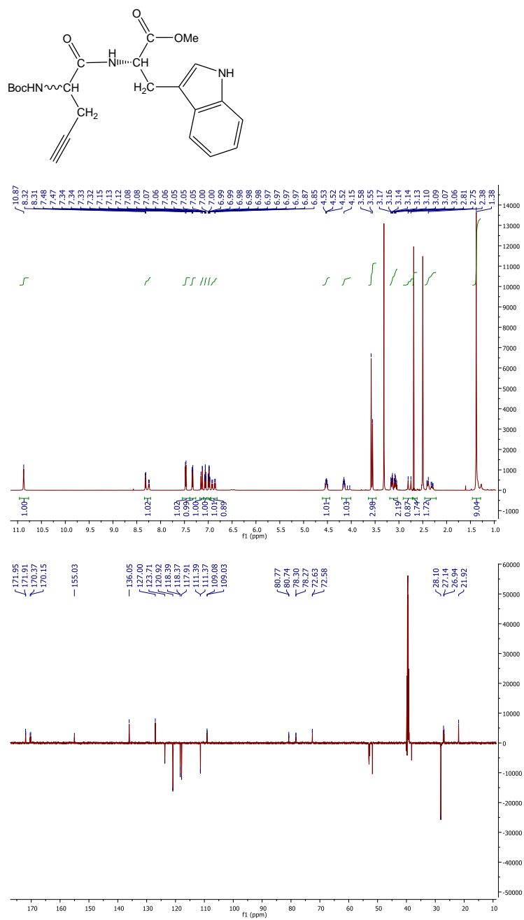
Slika D.8.3a. Struktura spoja 3 i ^1\text{H} NMR (600 MHz, DMSO- d_6 ), APT i spektri spoja 3 .
