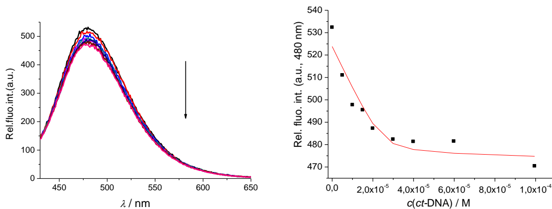
Slika D.8.15.a Fluorimetrijska titracija spoja 7 ( c = 5 \times 10^{-6} \text{ mol dm}^{-3} ; \lambda_{\text{exc}} = 352 \text{ nm} ) s ct -DNA (lijevo); Ovisnost intenziteta emisije pri \lambda_{\text{max}} = 480 \text{ nm} o c (polinukleotid), izračunato prema Scatchardovoj jednadžbi (pH = 7,0 u natrijevom kakodilatnom puferu, I = 0,05 \text{ mol dm}^{-3} ).
