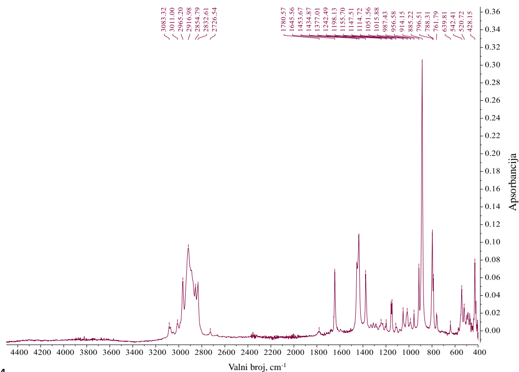
Slika 34. FTIR spektar komponente eteričnog ulja limonena
