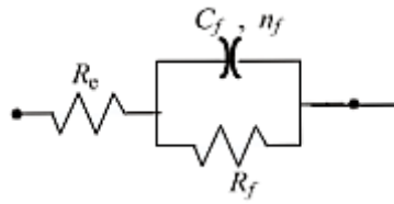
Slika 4.30. Ekvivalentni električni krug 1RC
