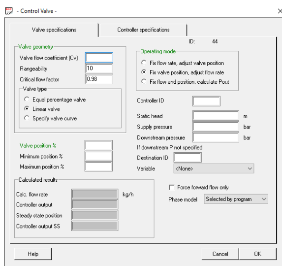
Slika 3.12. Definiranje regulacijskog ventila
