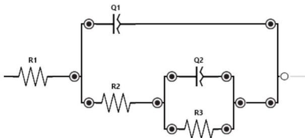
Slika 45: Električni ekvivalentni krug korišten u računalnom programu PStace 5.7. za prilagodbu EEK mjernim podacima
