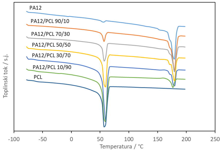
Slika 24. DSC termogram ciklusa zagrijavanja ishodnog PA12 i PCL i PA12/PCL mješavina
