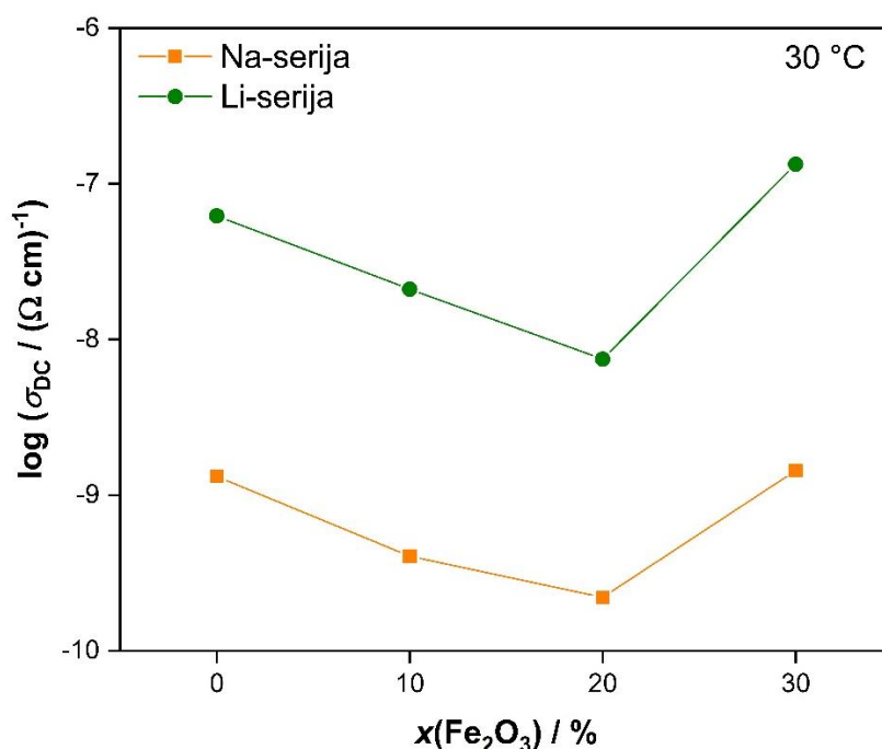
Slika 37. Ovisnost istosmjerne (DC) provodnosti na 30 °C o množinskom udjelu \text{Fe}_2\text{O}_3 za uzorke iz Na-serije i Li-serije stakala
