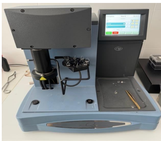
Slika 20. Termogravimetar TA Instruments Q500
