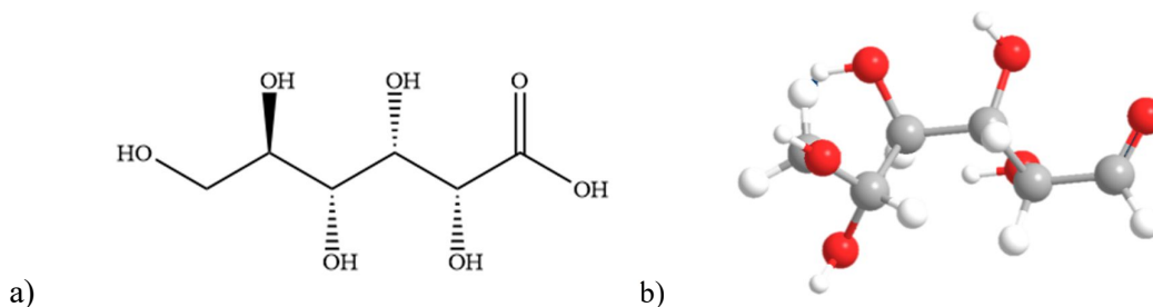
Slika 2. a) Kemijska struktura i b) 3D prikaz molekule glukonske kiseline
