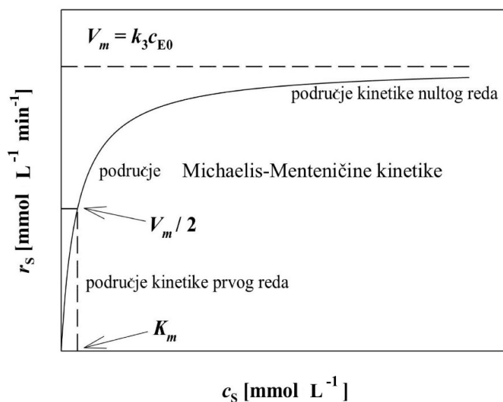
Slika 6. Ovisnost brzine reakcije o koncentraciji supstrata za Michaelis-Menteničinu kinetiku
