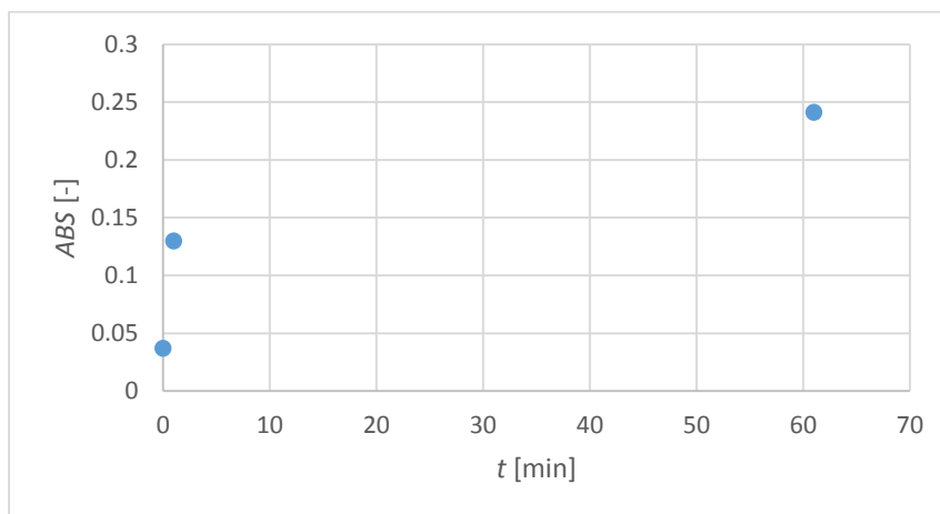
Slika 21. Sinteza Au nanočestica (redistirana voda, c(\text{K}_2\text{CO}_3) = 1 \text{ mM} , T = 37 \text{ }^\circ\text{C} , 150 \text{ rpm} , c_{\text{ureaze}} = 2 \text{ mg cm}^{-3} , c(\text{HAuCl}_4) = 4 \text{ mM} , V = 10 \text{ cm}^3 ), A) vremenska promjena koncentracije proteina, B) UV spektar, C) vremenska promjena apsorbanije dobivenog pika na UV spektru (455 nm)
