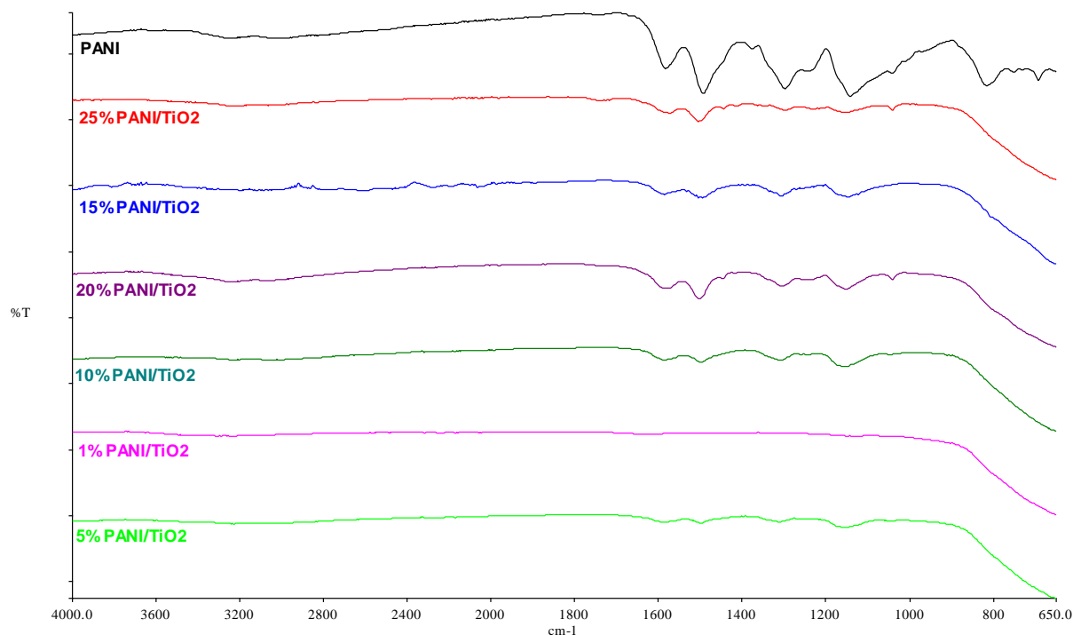
Slika 19. FTIR spektri čistog PANI-a i sintetiziranih nanokompozita PANI/TiO 2
