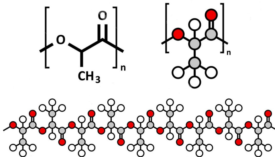
Slika 11. Struktura PLA [19]
