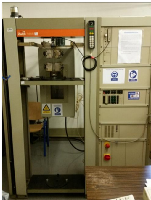
Slika 34. Mehanička kidalica Zwick 1445
