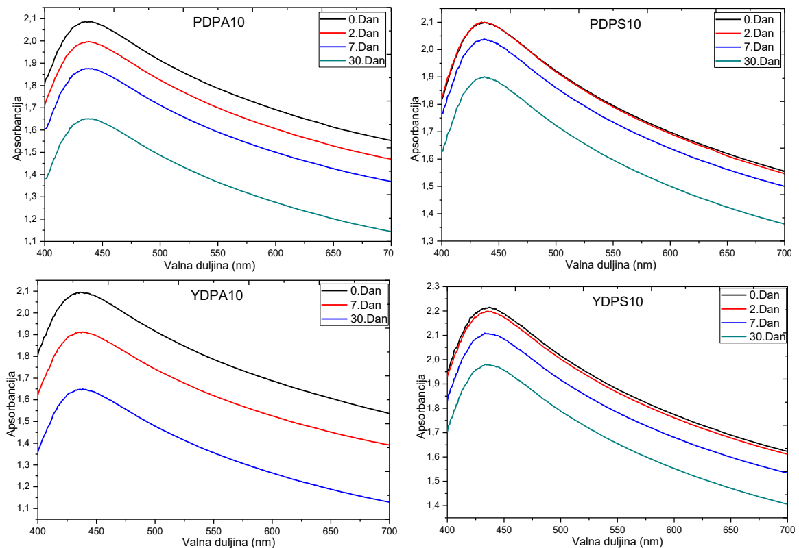
Slika 4.2.16. Promjena apsorbancije s vremenom sedimentiranja za sustave PAO4 / YUBASE4 + PAT + MWCNT
