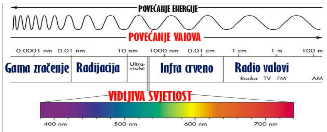
Slika 2.8. Elektromagnetski spektar
