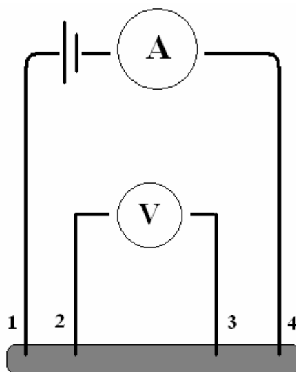
Slika 2.10. Shematski prikaz metode četiri točaka ( Four point probe)
