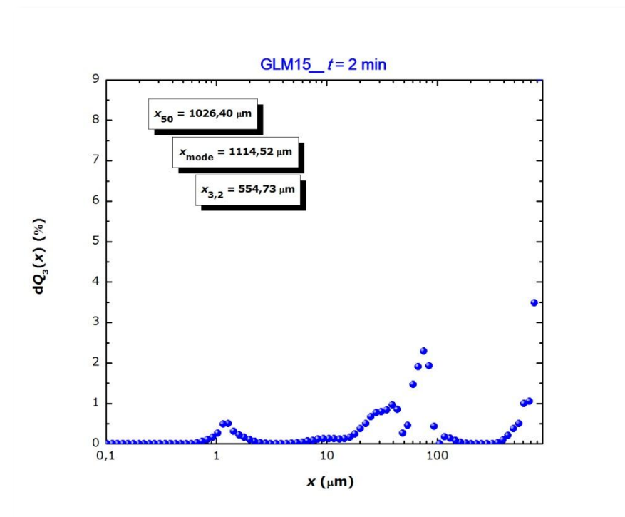
Slika 4.16. Grafički prikaz eksperimentalne raspodjele veličina čestica pomoćne tvari u kolektivu pri vremenu t = 2 min.
