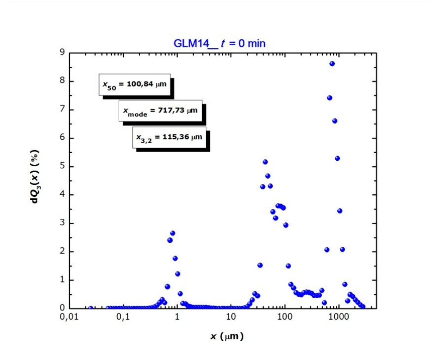
Slika 4.15. Grafički prikaz eksperimentalne raspodjele veličina čestica pomoćne tvari u kolektivu pri vremenu t = 0 min.
