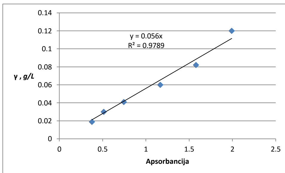
Slika 4.2.3. Baždarni pravac međuovisnosti masene koncentracije čestica grafena u PAO ulju i apsorbanca u UV/VIS području
