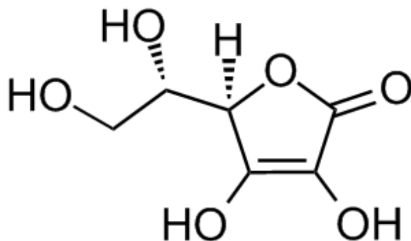
Slika 1. Struktura L-askorbinske kiseline, \alpha -ketolaktona molekulske formule \text{C}_6\text{H}_8\text{O}_6 i molekulske mase 176,13
