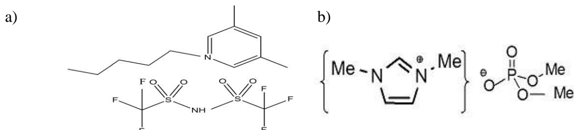
Slika 3.1. Primjer struktura ionskih kapljvina: a) [hmppy][NTf 2 ] kojoj je kationska baza N-alkil piridinijev kation b) [mmim][DMP] kojoj je kationska baza N-alkil imidazolijev kation 8
