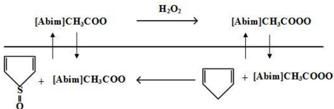
Slika 3.6. Mehanizam oksidacijske desulfurizacije ionskim kapljevina [\text{Abim}]\text{CH}_3\text{COO} (A-alkilni supstituent) uz oksidans \text{H}_2\text{O}_2 10
