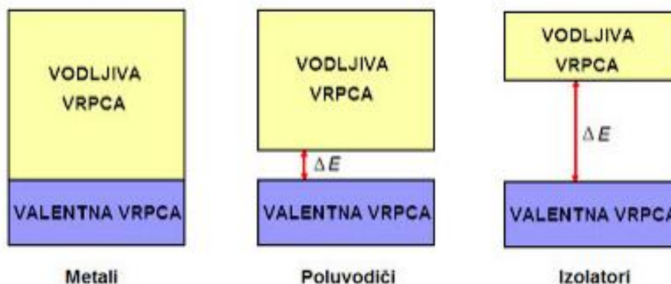
Slika2.13. Vodljiva i valentna vrpca te zabranjena zona
