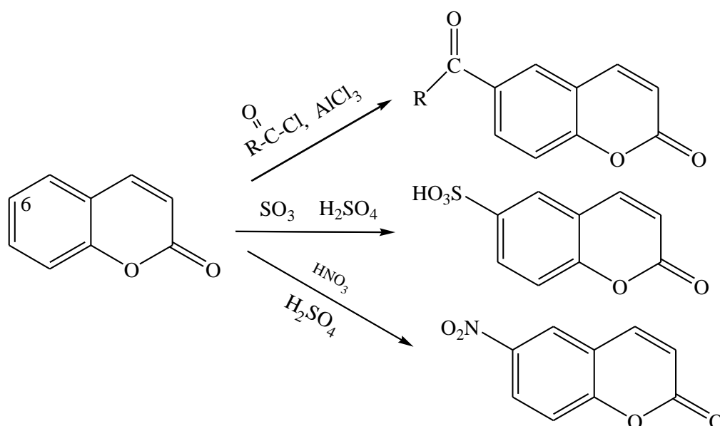
Shema 3. Elektrofилна supstitucija (nitriranje, sulfoniranje i Friedel-Crafts-ovo aciliranje) na kumarinu
