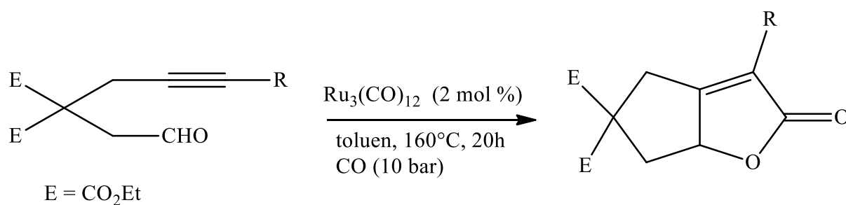
Shema 12. Primjer domino reakcije
