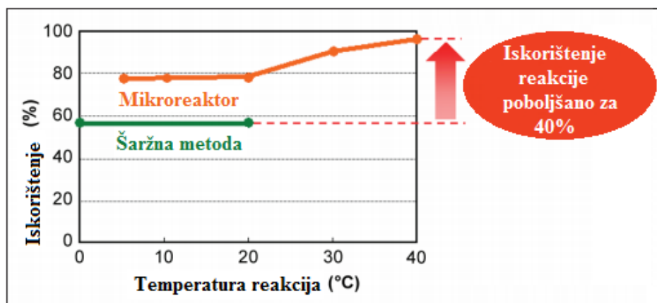
Slika 17. Ovisnost iskorištenja reakcije u ovisnosti o temperaturi reakcije [2]
