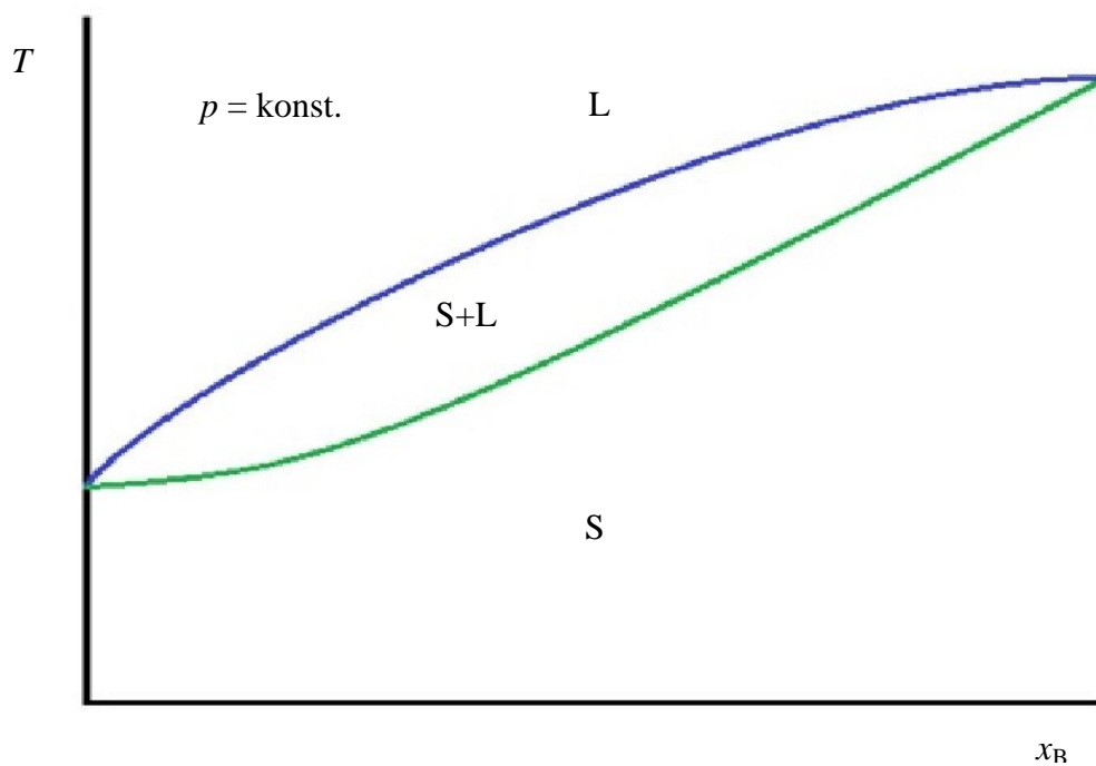
Slika 2.3 Fazni dijagram za ravnotežu krutina-kapljevina gdje su komponente potpuno mješljive u kapljevitoj i krutoj fazi.
