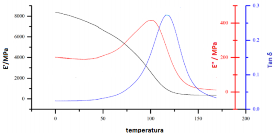
Slika 4. DMA termogram
