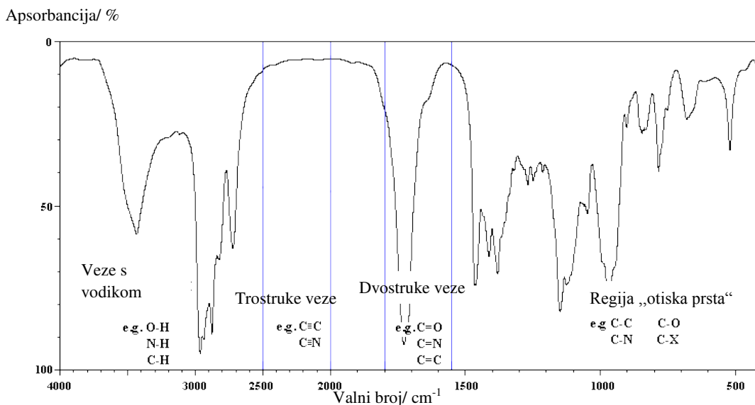
Slika 27. FTIR spektar s tipičnim područjima signala
