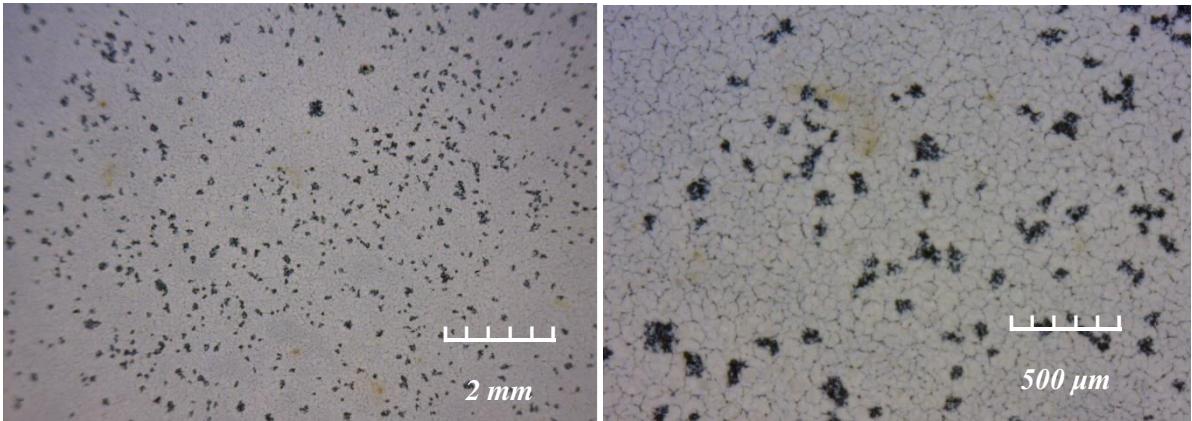
Slika 48. Uzorak NTD2 nakon odljepljivanja ljepljive trake pri uvećanju od 60x (lijevo) i 200x (desno)
