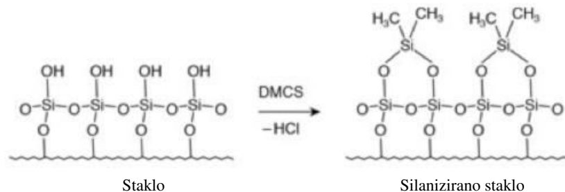
Slika 23. Struktura površine stakla prije i nakon aktivacije silanom u kiselom mediju
