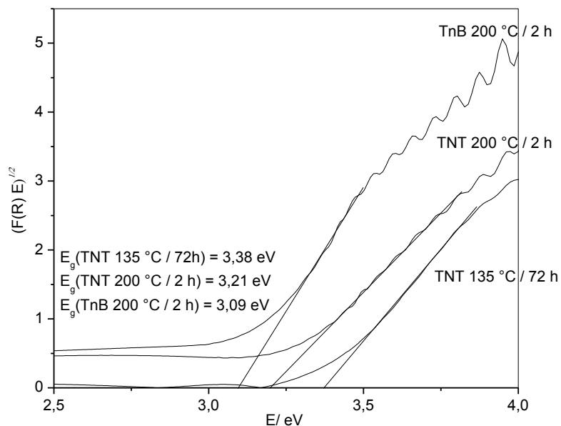
Slika 67. Taucov grafički prikaz za titanatne nanocjevčice i TnB prije i nakon termičke obrade
