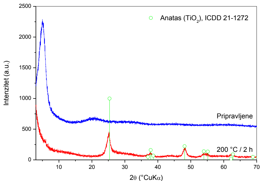
Slika 58. Difraktogram TnB prije i poslije termičke obrade na 200 °C u trajanju od 2 h
