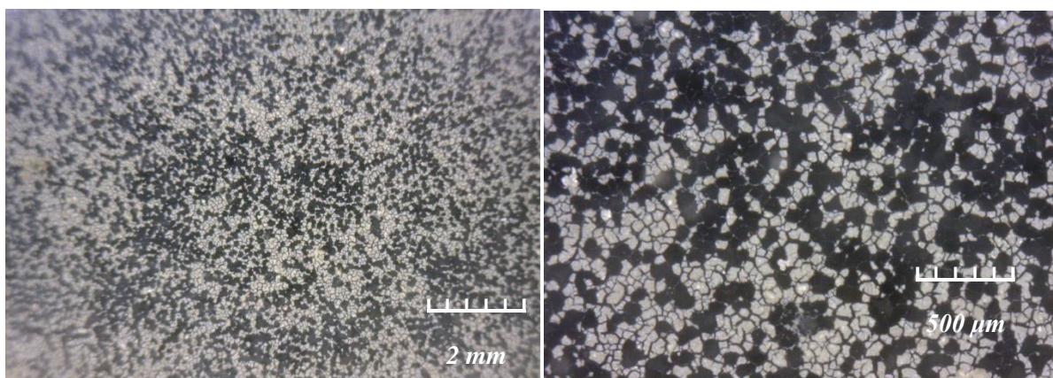
Slika 52. Uzorak NTD4 nakon odljepljivanja ljepljive trake pri uvećanju od 60x (lijevo) i 200x (desno)
