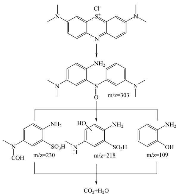
Slika 18. Shematski prikaz stupnjevitog raspada molekule metilenskog modrila
