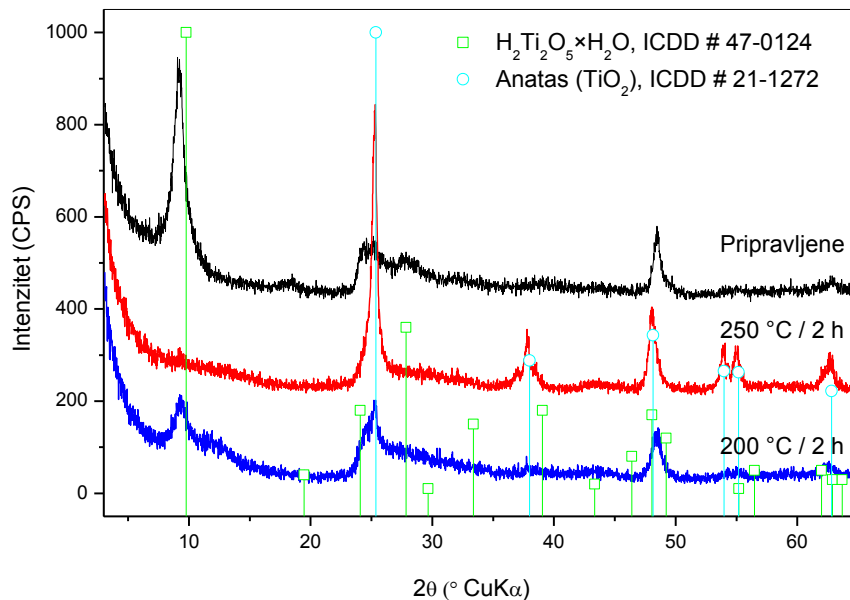
Slika 57. Difraktogram titanatnih nanocjevčica prije i poslije termičke obrade na 200 i 250 °C u trajanju od 2 h
