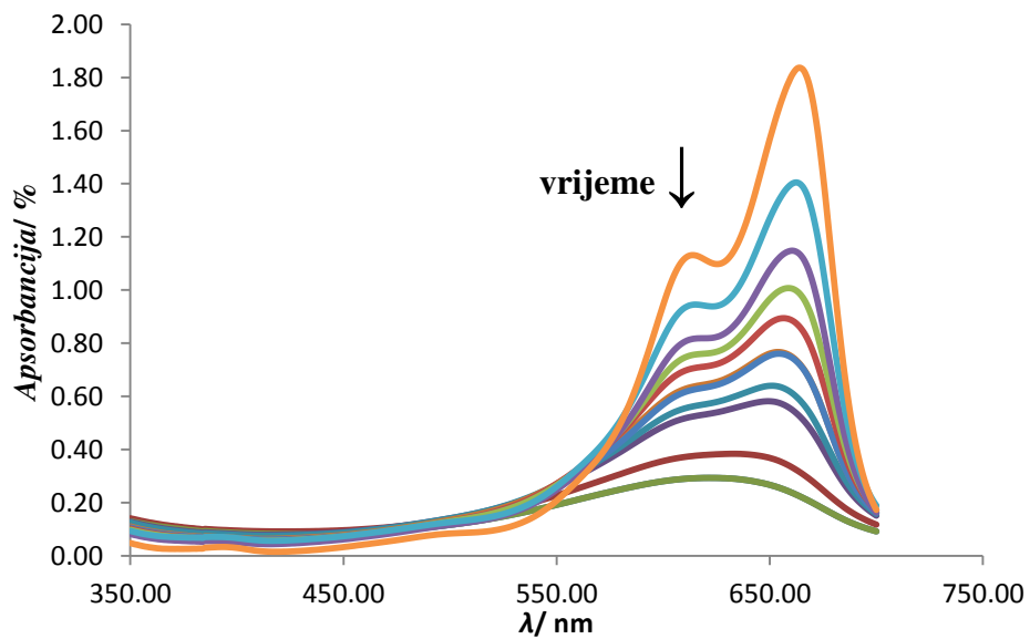
Slika 72. UV-Vis spektri metilenskog modrila nakon degradacije u prisutnosti uzorka NTD4
