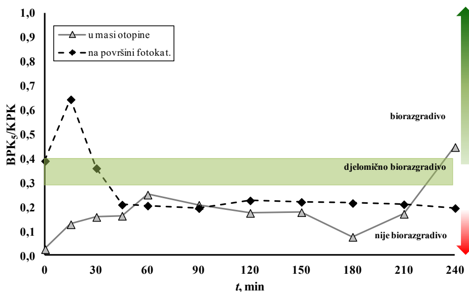
Slika 20. Promjena vrijednosti omjera BPK 5 /KPK tijekom fotokatalitičke razgradnje otopine DCF-a.
