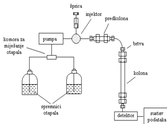
Slika 4. Shema rada HPLC-a.
