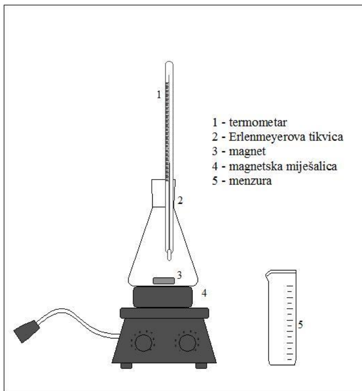
Slika 3.1. Aparatura za oksidaciju DAS-a vodikovim peroksidom ( H_2O_2 ) u ledenoj octenoj kiselini ( CH_3COOH ) te u N-metil pirolidonu ( C_5H_9NO )
